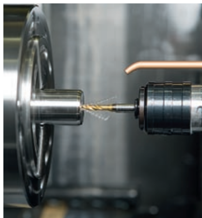
Axiale tapgatbewerking
